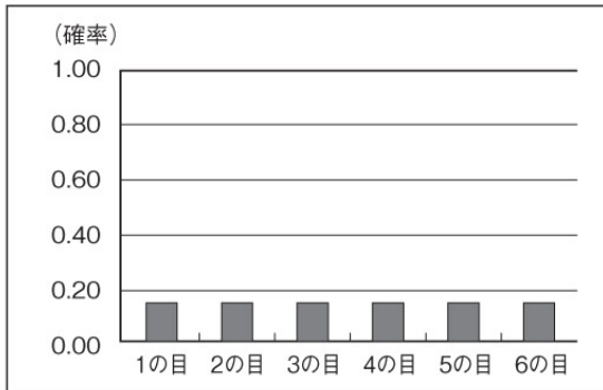
図3-2 サイコロを一回振ったときに出る目の確率分布図
